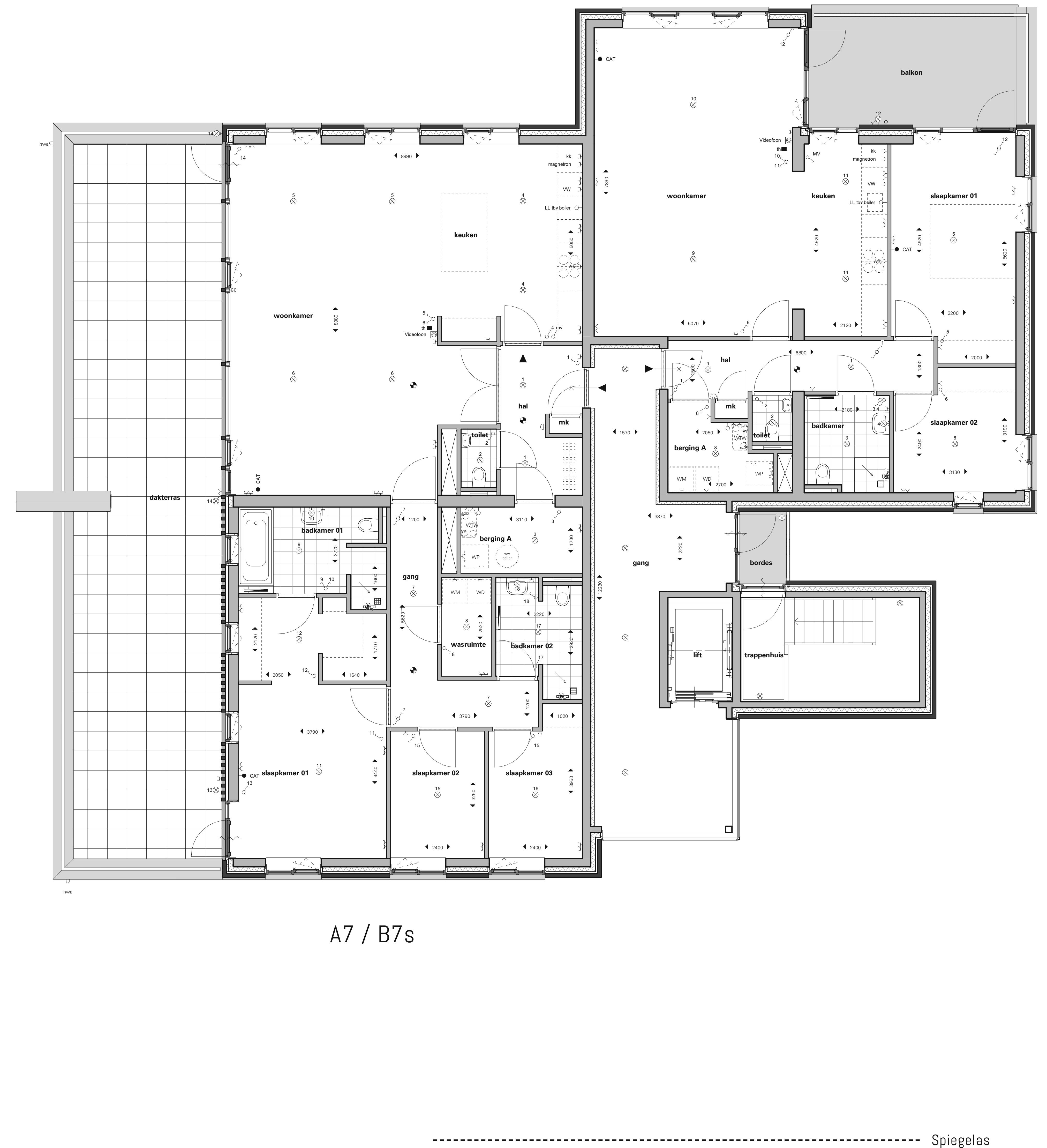
Tweede verdieping blok A Blok B is gespiegeld over "spiegelas"
